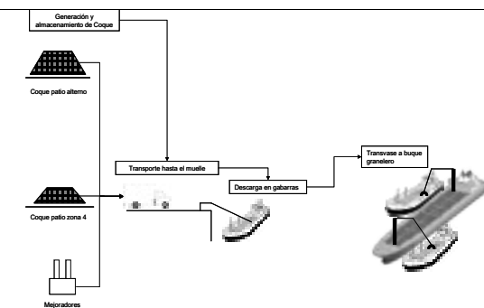
Ingeniería para Adecuar el Atraque Lateral de Gabarras en la Plataforma del Muelle de Servicios de Petroanzoátegui ENERGY COAL DE VENEZUELA Estado Anzoátegui. Venezuela Ingeniería de Detalle
